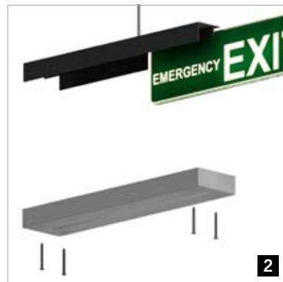
Scheibenpaar wird seitlich eingeschoben
